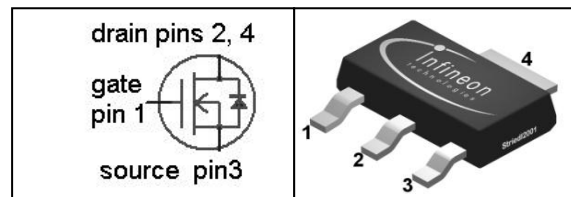
PG-SOT223
