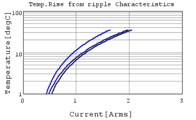
GCM31MR71H684KA55 Temp.rise — 200kHz
