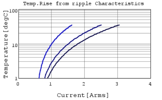
GRM188R61A474KA61 Temp.rise — 200kHz —
