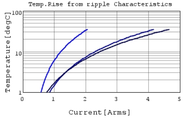
GRM219R61A105KA01 Temp.rise — 100kHz —
