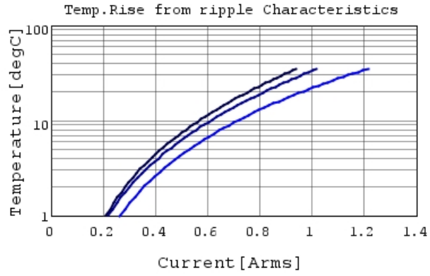
GRM1555C1H620JA01 Temp.rise — 200MHz
