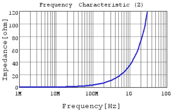
LQW15AN5N6G80 |Z|
