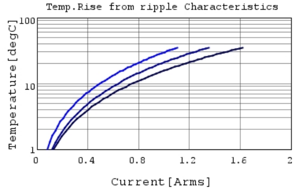
GRT155C81E224KE01 Temp.rise — 300kHz
